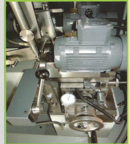
Talaş miktarı takibi için dahili komparatör Dial gauge to follow the infeed amount Количество фишек для внутреннего контроля
